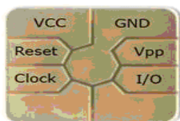
قسمت‌های مختلف محل‌های تماس کارت‌های هوشمند با کارت‌خوان
